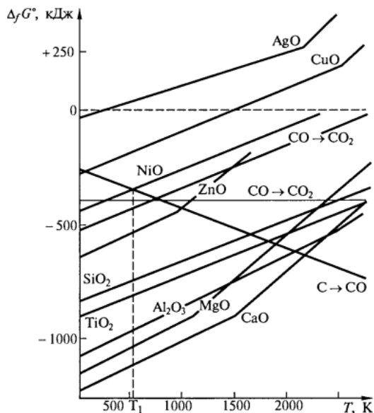
Пример диаграммы Эллингхэма для восстановления оксидов металлов
